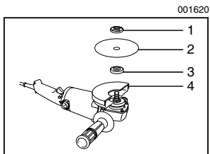
1. Contratuera 2. Disco de corte abrasivo 3. Brida interior 4. Protector de disco para un disco de corte
